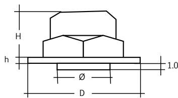
HEX NUT
