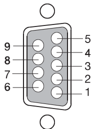
X2 D-sub socket 9-pin
