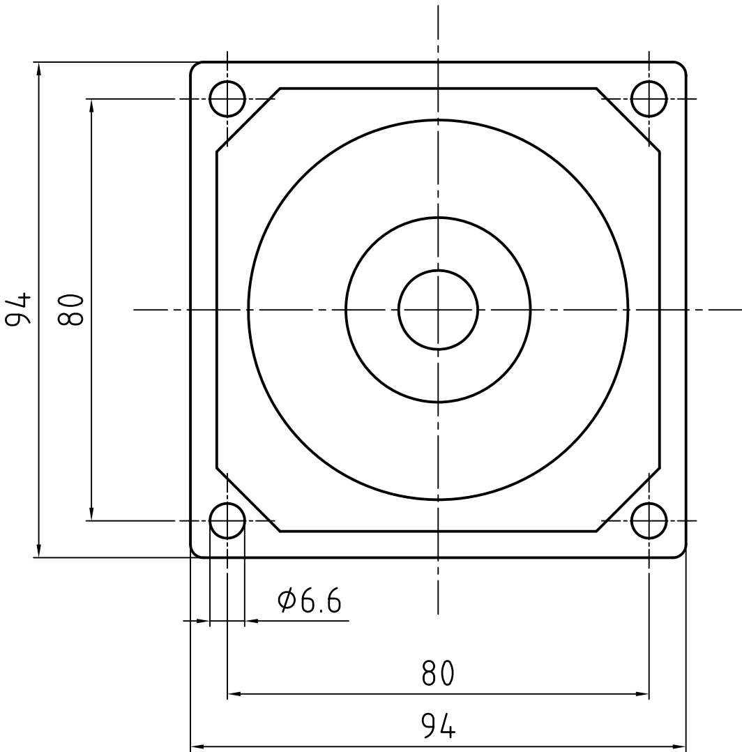
Ansicht A
